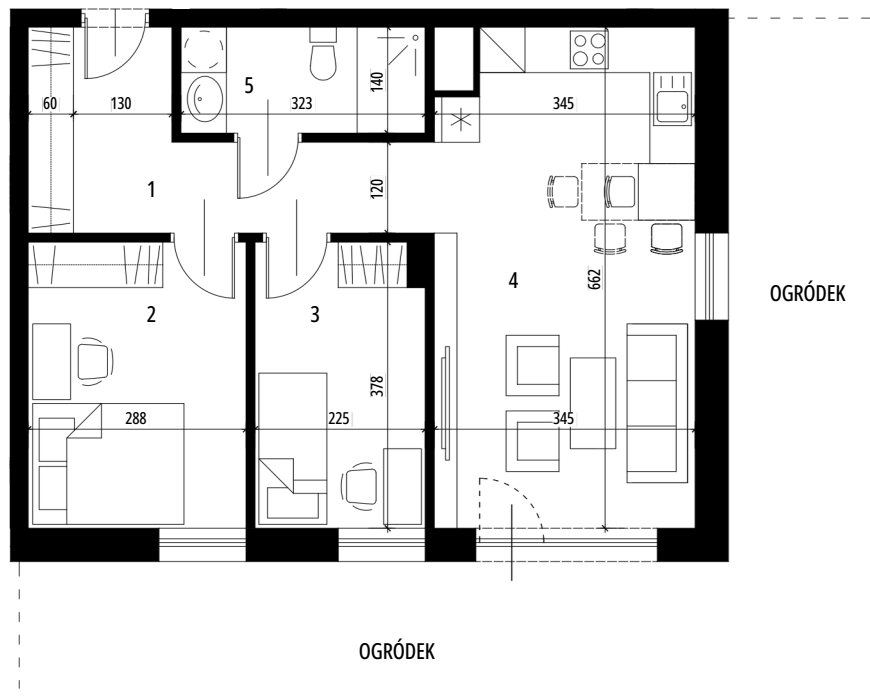
PLAN MIESZKANIA
