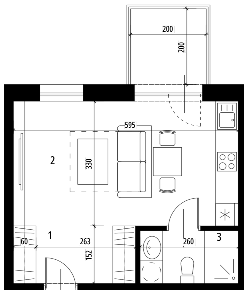
PLAN MIESZKANIA
