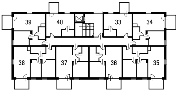
PLAN 4 PIĘTRA
