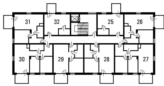
PLAN 3 PIĘTRA
