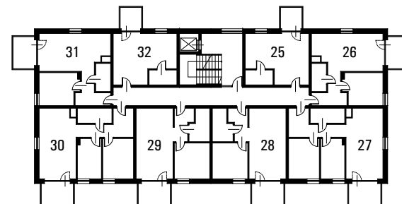
PLAN 3 PIĘTRA
