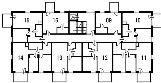
PLAN 1 PIĘTRA
