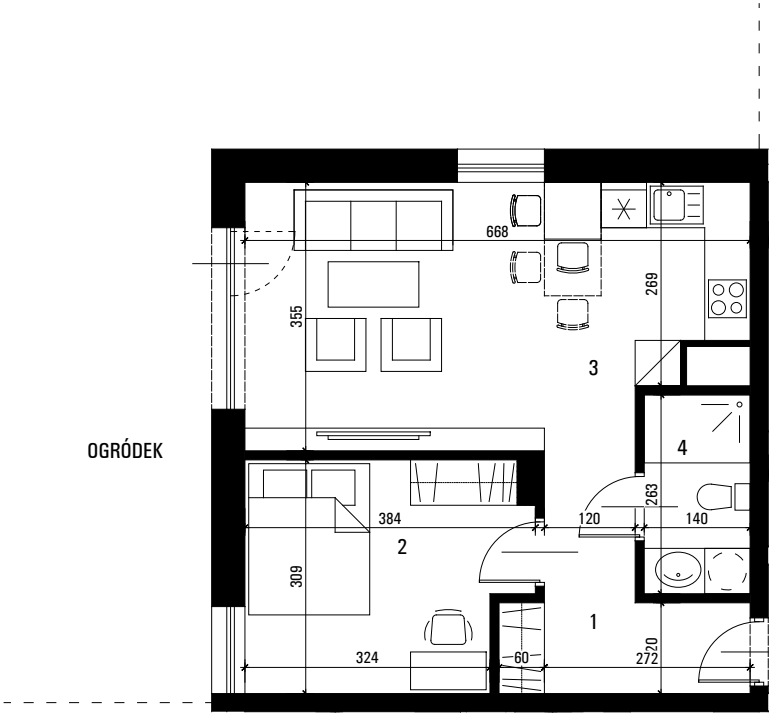
PLAN MIESZKANIA
