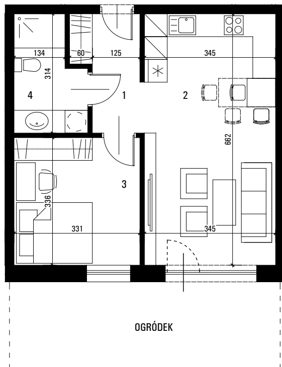
PLAN MIESZKANIA
